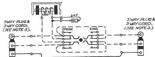
FIG.2. CORD CIRCUIT.
